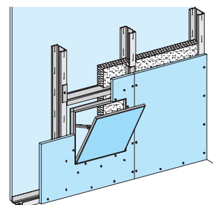
revizní klapka Knauf ALUTOP REVO
