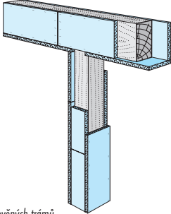
Opláštění dřevěných trámů
