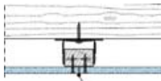
Fugenkleber Spára < 1 mm (odstraňte vytlačené lepidlo)
