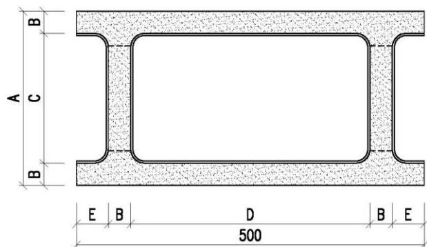
TABULKA ROZMEROV
